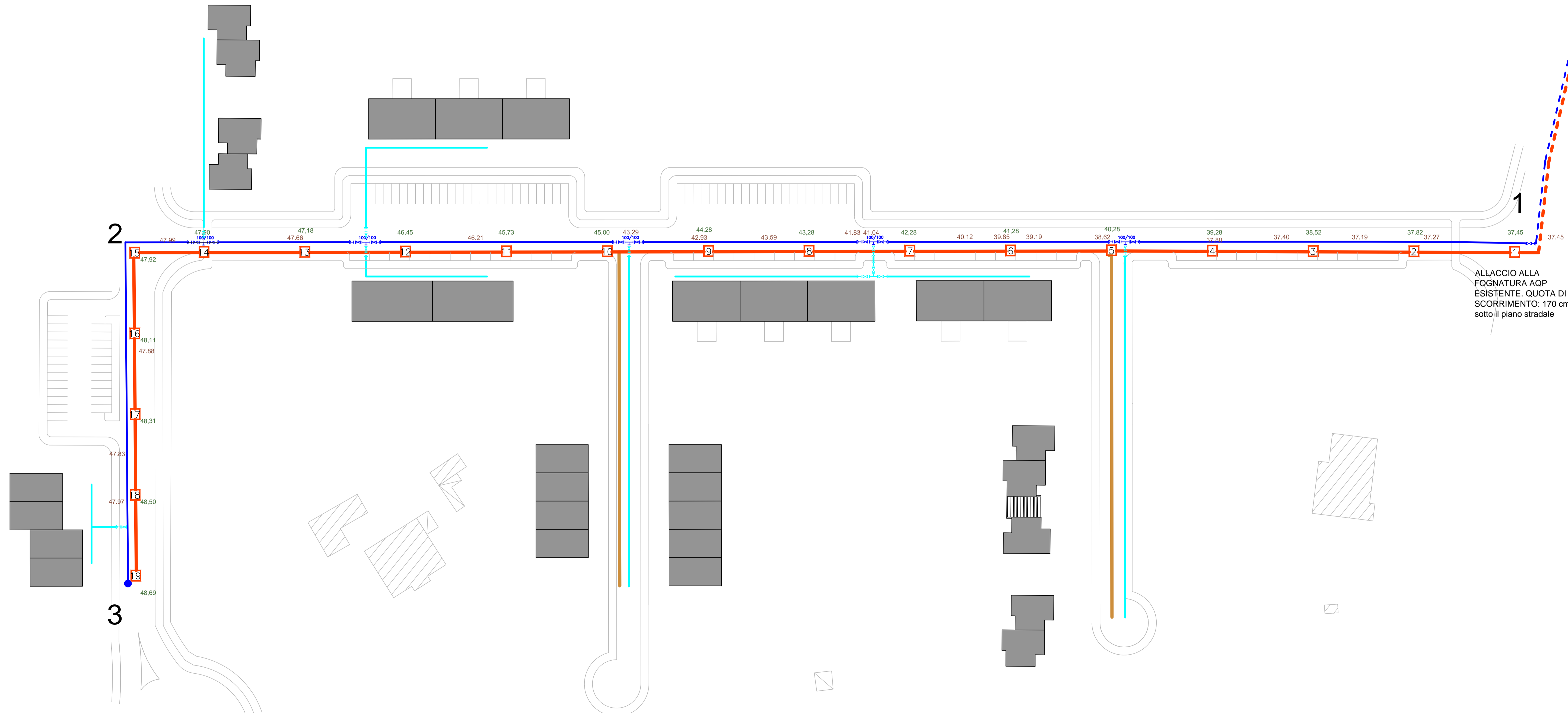
PLANIMETRIA QUOTATA DI PROGETTO RETE DI FOGNATURA TRONCO 1-2 scala 1:500
