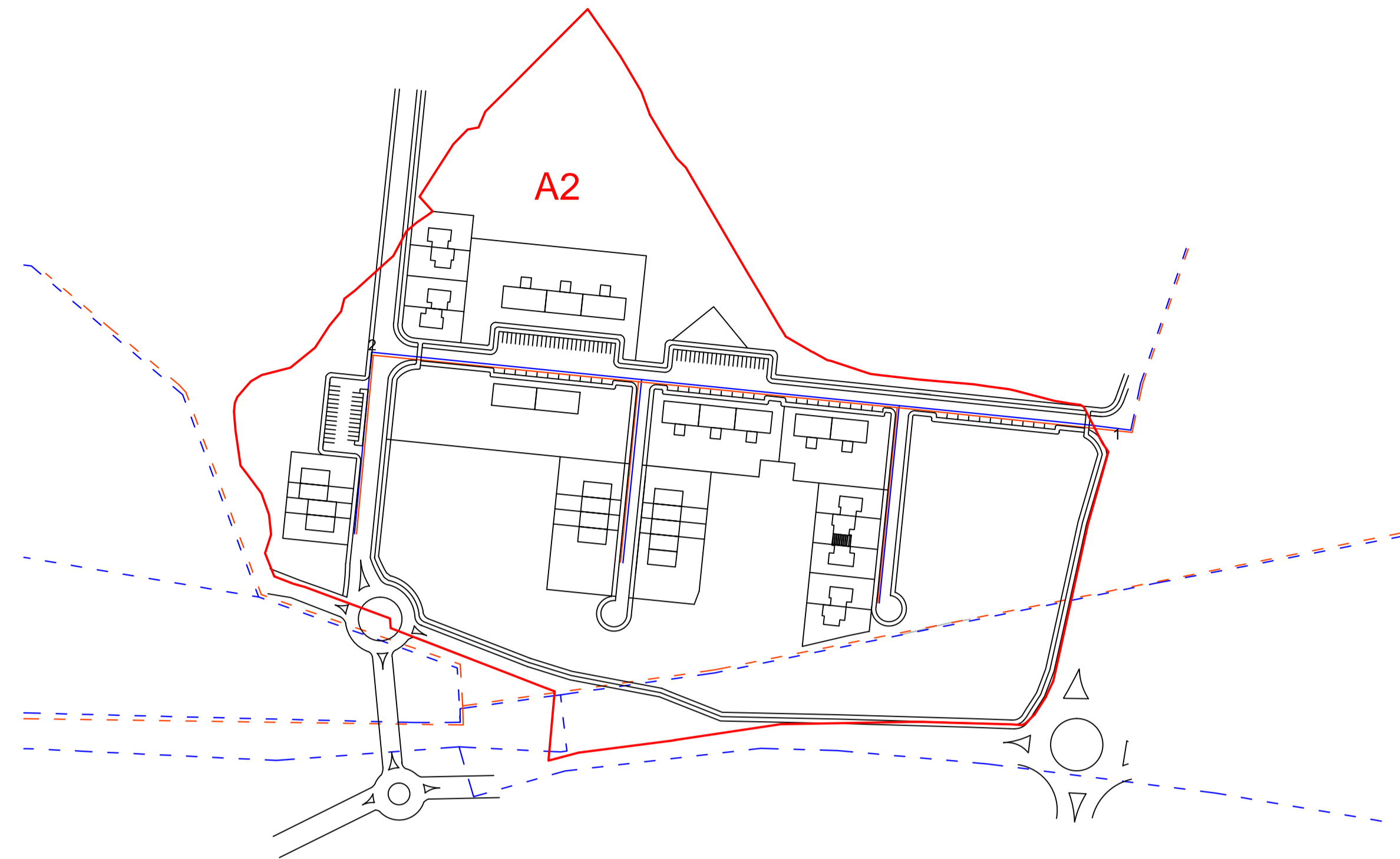
PLANIMETRIA QUOTATA DI PROGETTO RETE DI FOGNATURA TRONCO 1-2 scala 1:500
