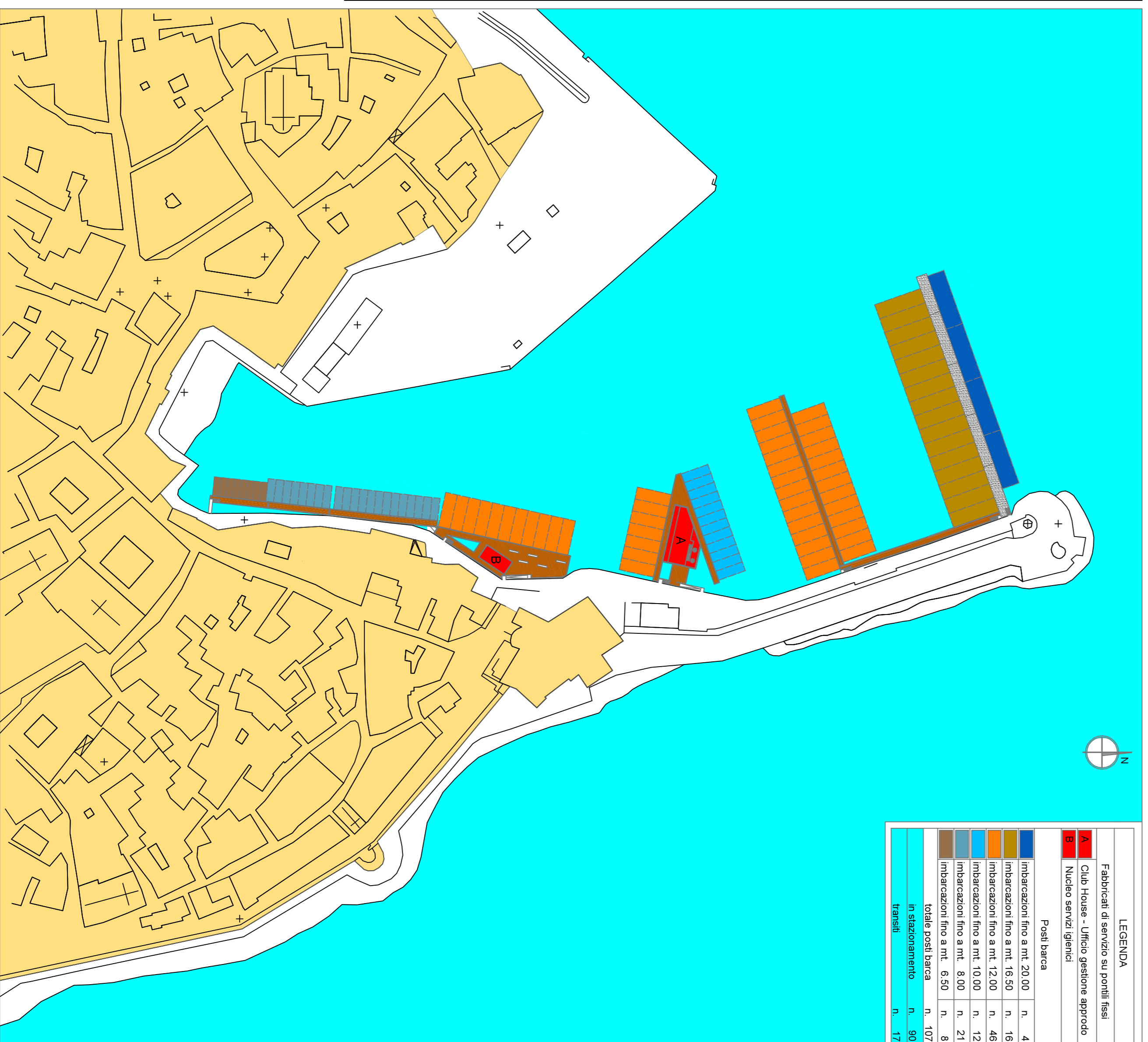
PORTO di MONOPOLI Progetto per un approdo turistico - Pianimetria generale d'intervento
