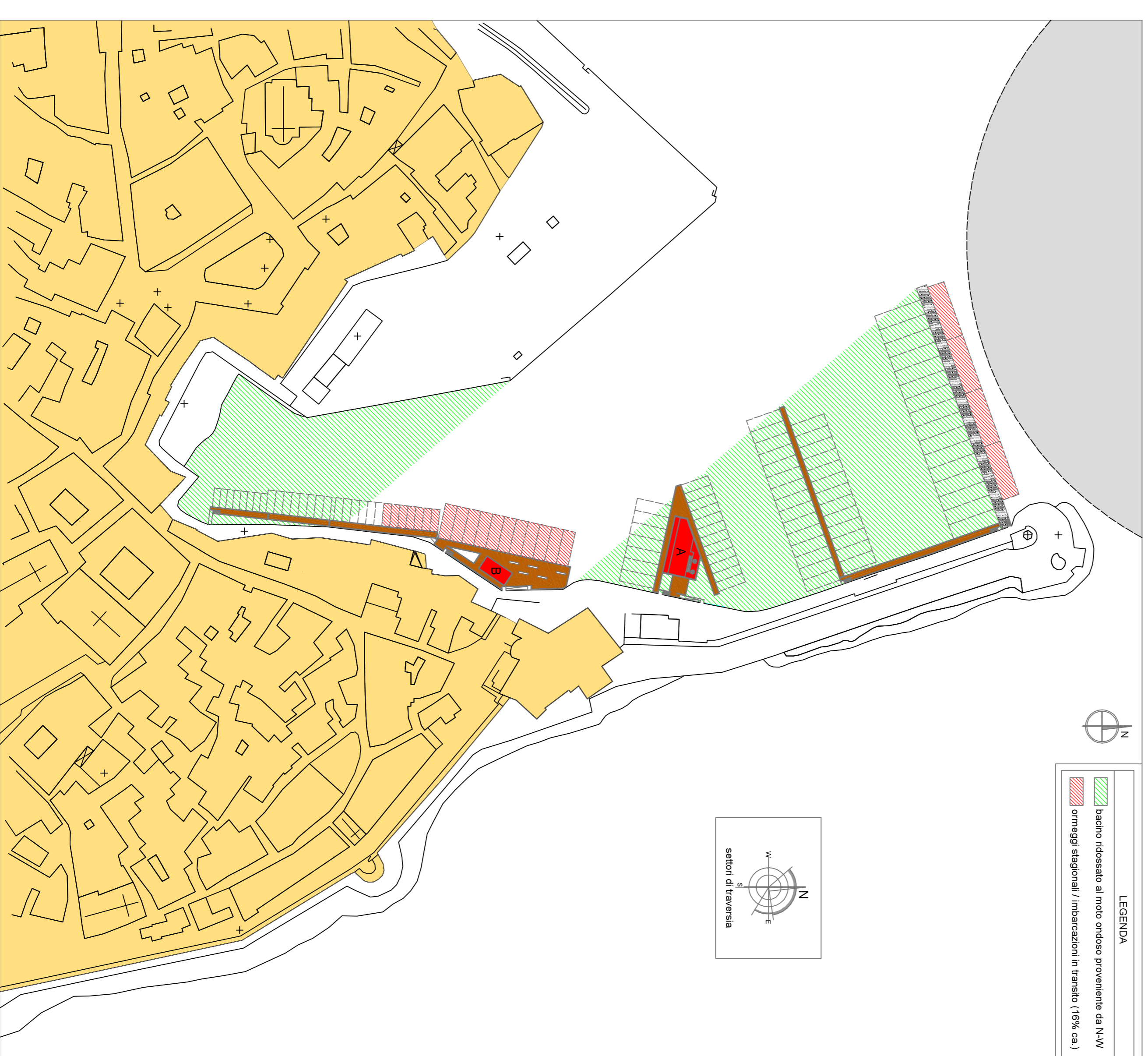
PORTO di MONOPOLI Progetto per un approdo turistico - Individuazione ridossi al moto ondosso proveniente da N-W - Individuazione ormeggi per stazionamento e stagionali / transiti
