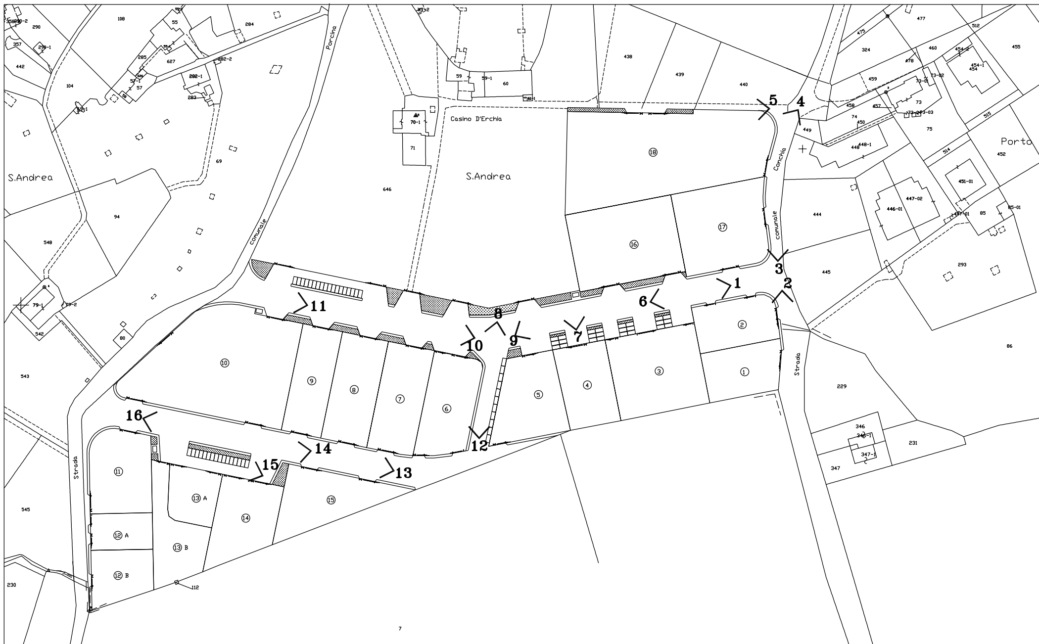
PLANIMETRIA CON INDICAZIONE DEI PUNTI DI PRESA
