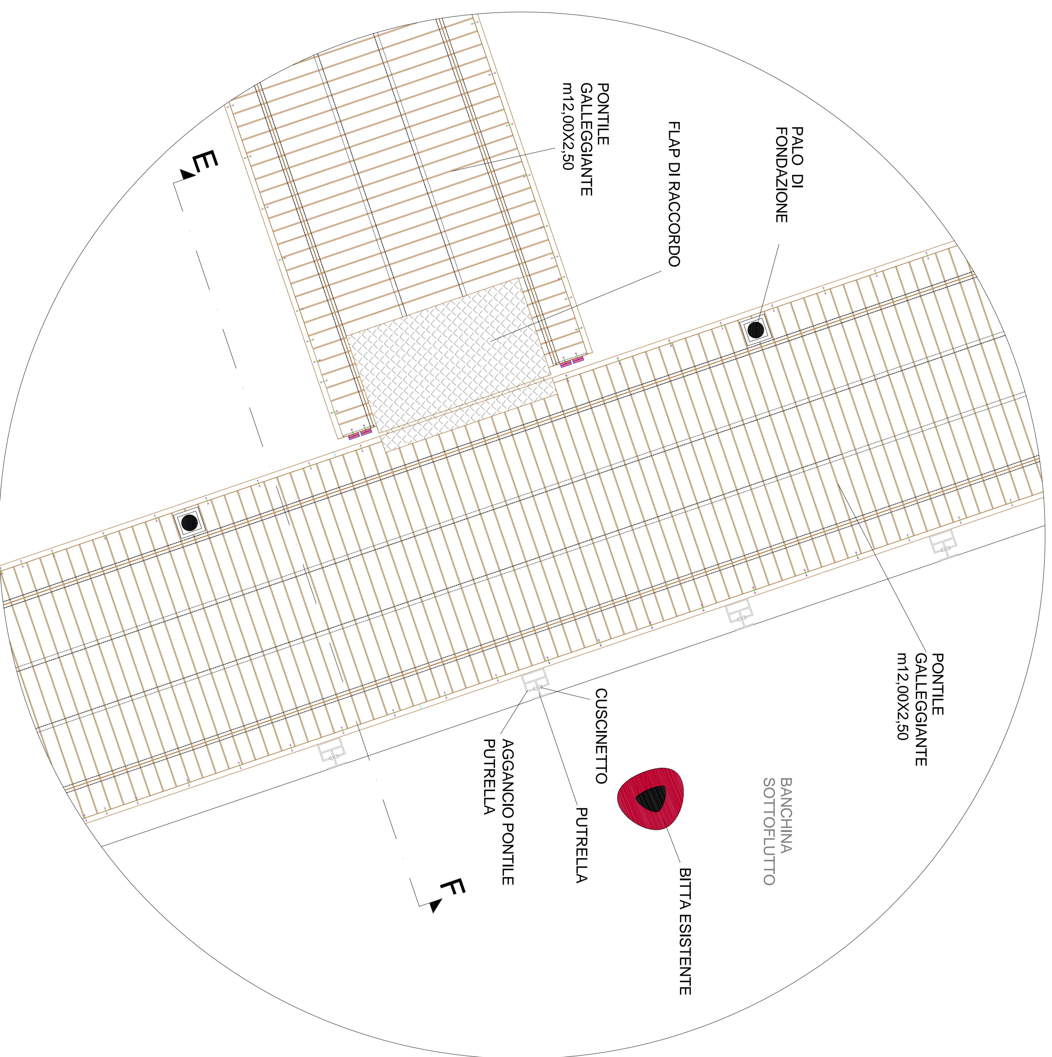
PIANTA SCALA 1:20
