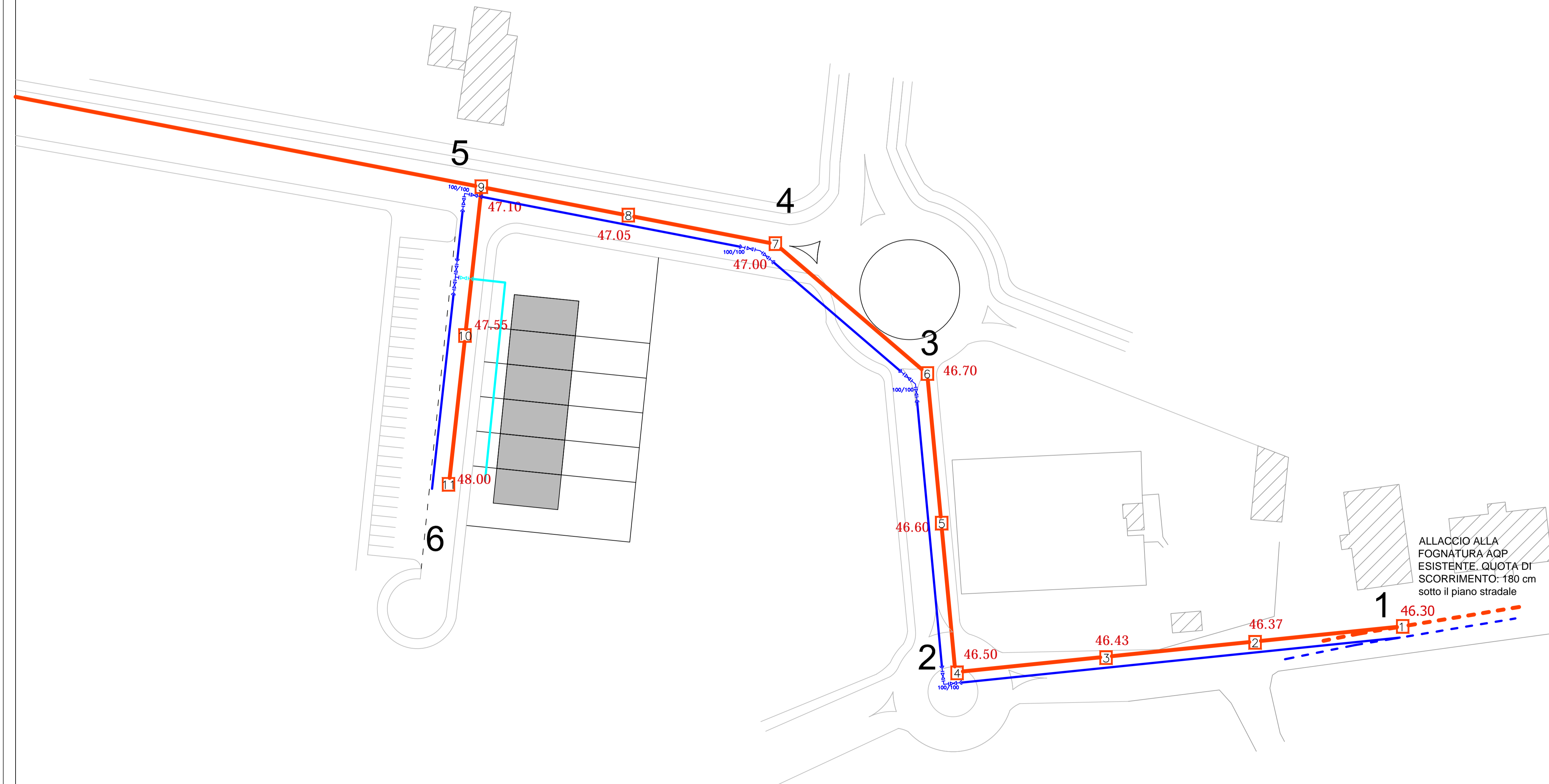
PLANIMETRIA QUOTATA DI PROGETTO RETE DI FOGNATURA TRONCO 1- 2-3 3-4 4-5 5-6 scala 1:500
